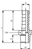
Einschraubschlauchtüllen, Außengewinde konisch
