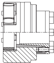
ROTEX® Nabe Ausf. 4.2 in Kombination mit CLAMPEX® KTR 250
