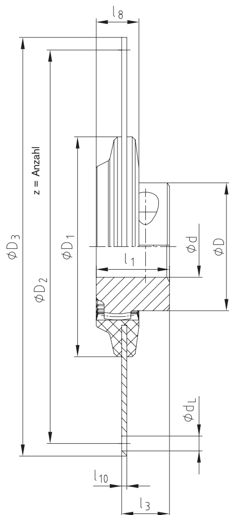
Anbau kurz
