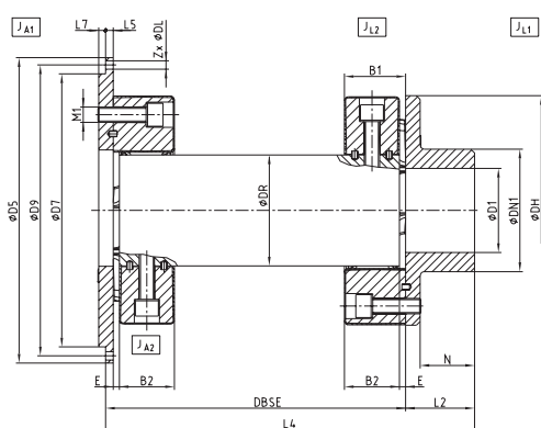
Größe 12 - 280
