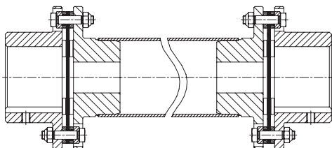
Bauart NNW (s. Seite 180)
