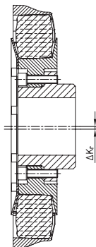
Radialverlagerung
