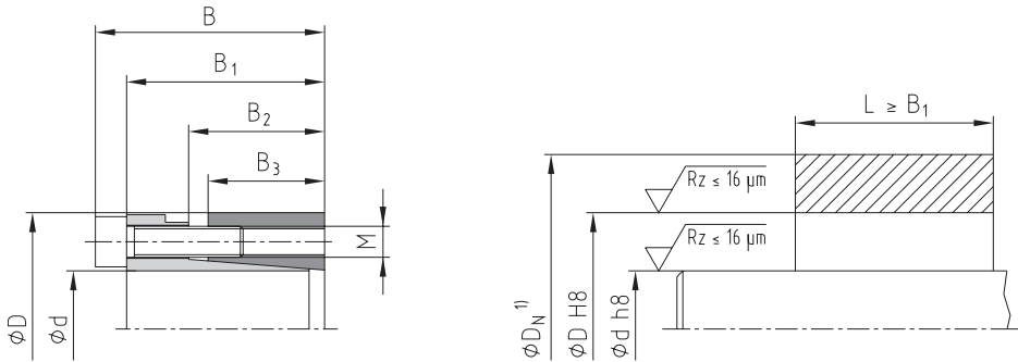
Anwendungsbeispiel Nabenform
