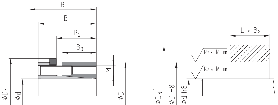
Anwendungsbeispiel Nabenform
