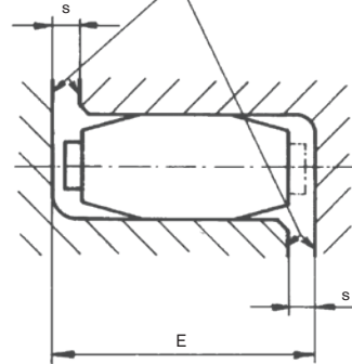
Elektrische Isolierung durch Spaltmaß „s“
