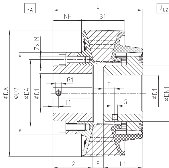
Verlagerungen – Bauart HEW Compact
