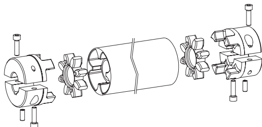
7.1 = SPLIT-Nabe mit Passfedernut
