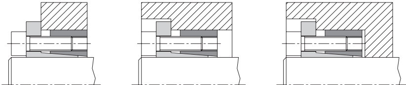
Anwendungsbeispiel Nabenform
