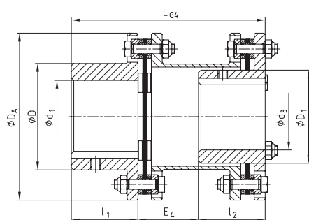
Bauart NENA 1
