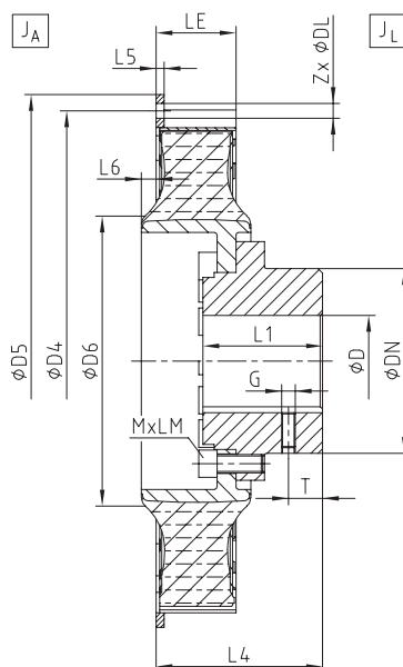
Bauart AL
