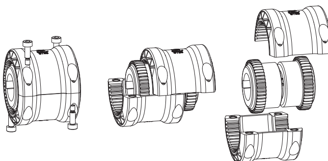
BoWex® Bauart GT mit geteilter Hülse
