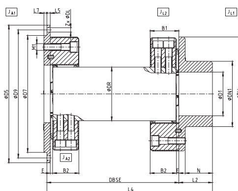
Größe 360 - 560
