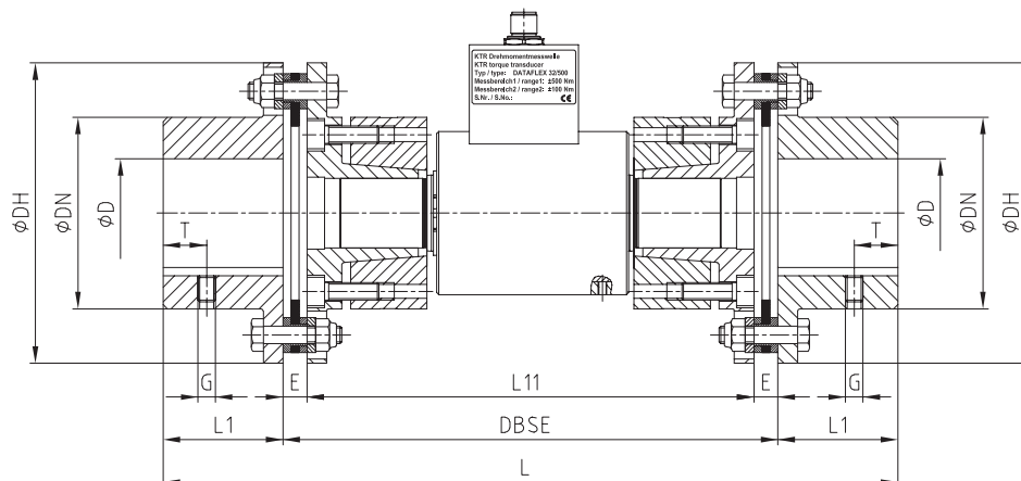
Abmessungen [mm] der Drehmomentmesswelle und der Kombination mit RADEX®-NC Nabenausführung, 3.5 Kupplungen
