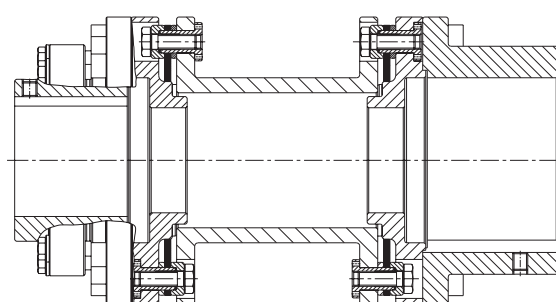
RIGIFLEX®-N mit integrierter Rutscheinheit siehe Maßblatt 698869
