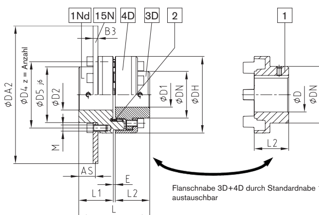
Bremsscheibe Bauart ADR-SBA
