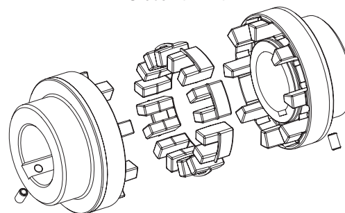
Größe 140 - 280
