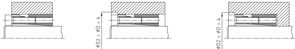
Anwendungsbeispiel Nabenform
