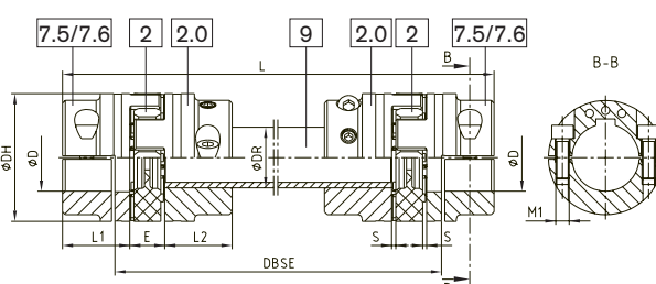
Bauart ZR (mit GS-Zahnkranz und DH-Klemmnaben für doppelkardanische Verbindung 7.5 oder 7.6) 3)
