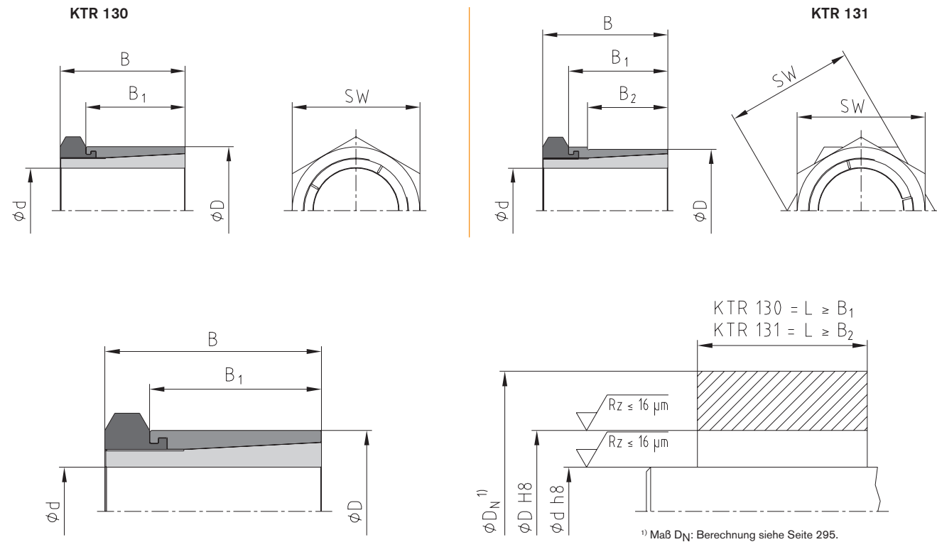
Anwendungsbeispiel Nabenform
