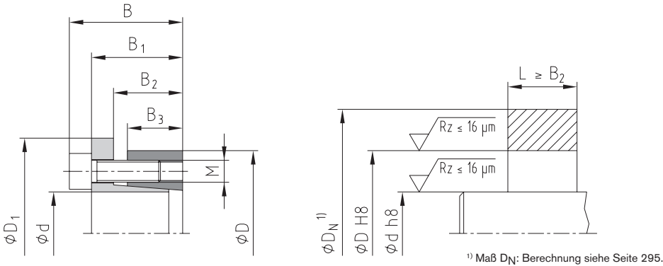
Anwendungsbeispiel Nabenform
