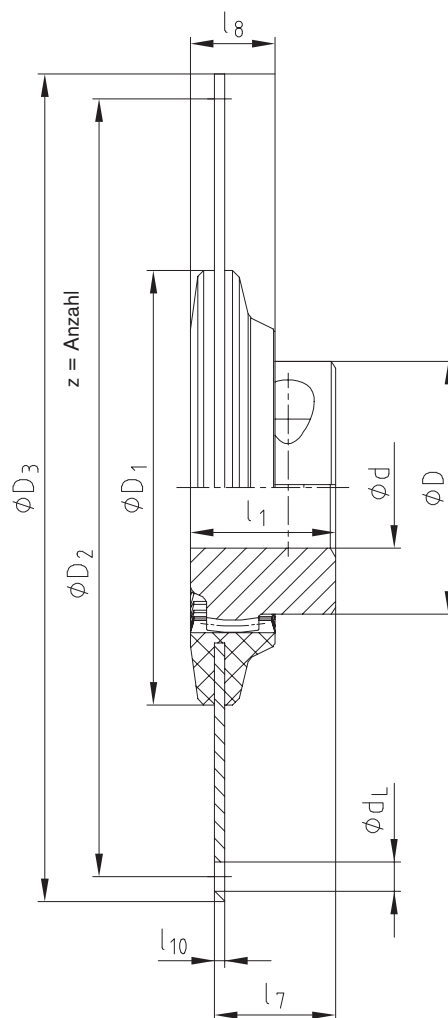
Anbau lang
