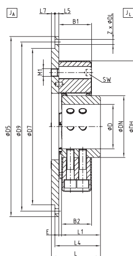
Größe 360
