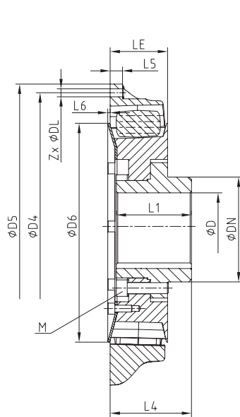
Ausführung A (direkter Flansanschluss)
