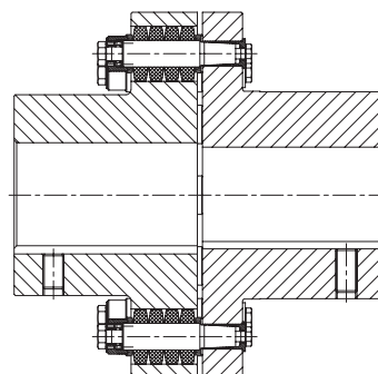
Spielfreie Ausführung
