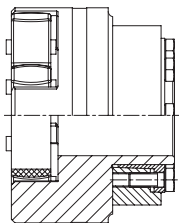
ROTEX® Nabe Ausf. 4.9 in Kombination mit CLAMPEX® KTR 620
