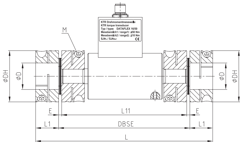
Kombination DATAFLEX® 16 mit RADEX®-NC
