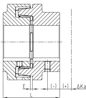
Axialverlagerung ΔK a
