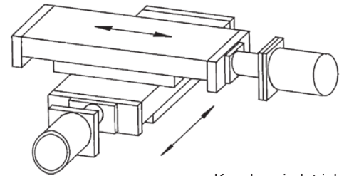
Kugelgewindetrieb
