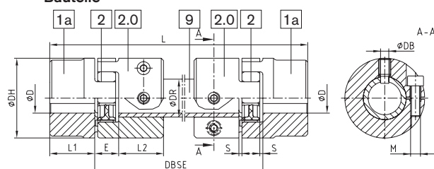
Bauart ZR (mit GS-Zahnkranz) 3)
