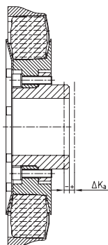
Axialverlagerung
