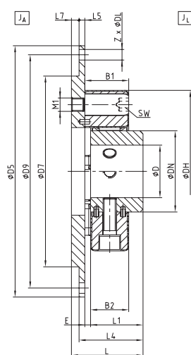
Größe 12 - 280
