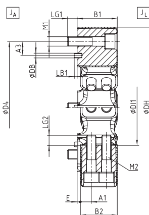
Größe 360 - 560
