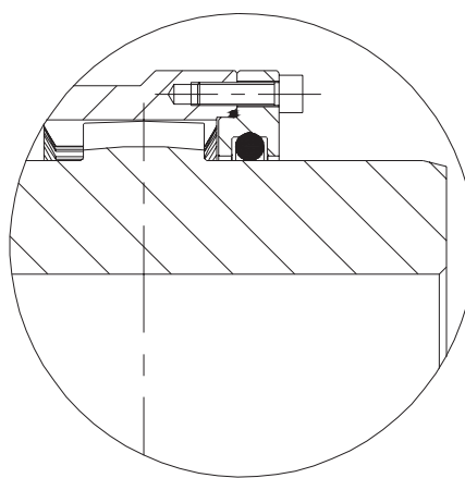
Bauart DH
