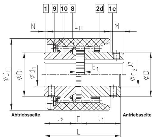
BoWex® Bauart Spez.-I/CD
