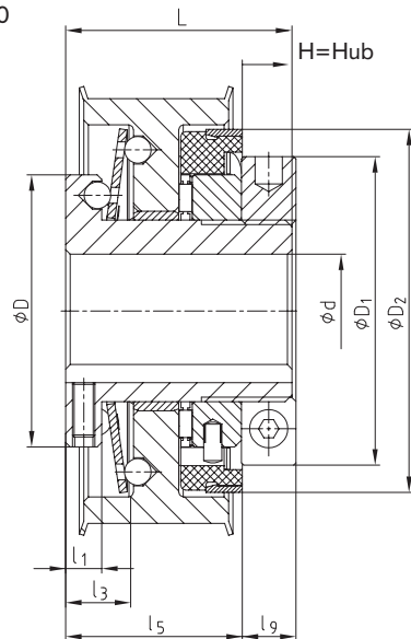
Nabenausführung 1.0
