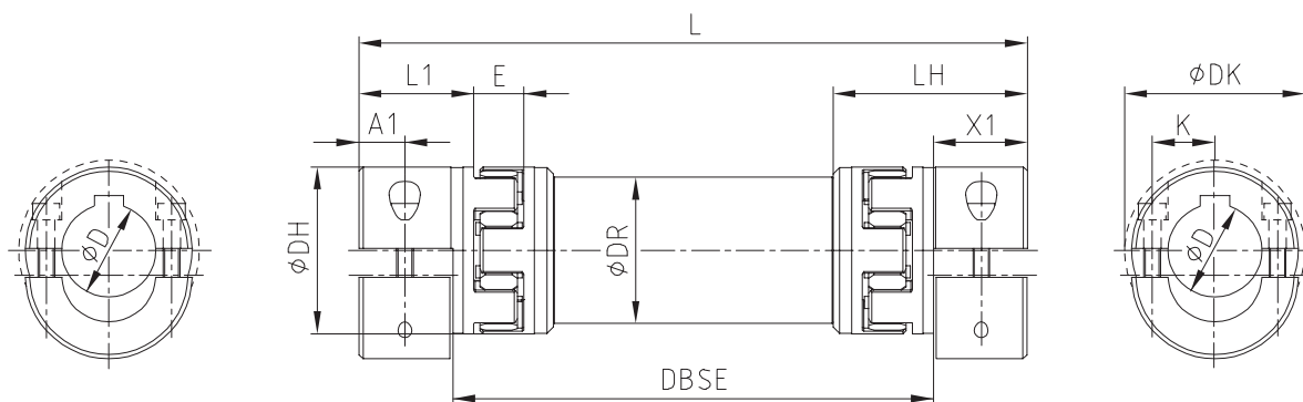
Wellenabstandsmaß
