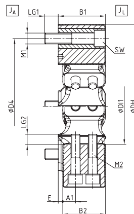
Größe 560
