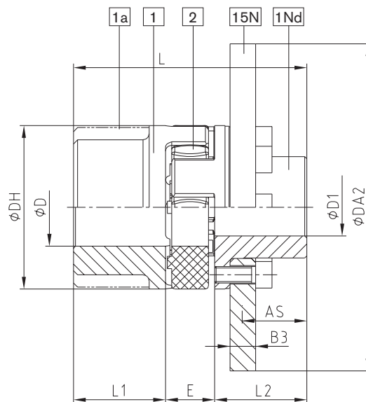
Bremsscheibe Bauart SBAN
