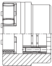
ROTEX® Nabe Ausf. 4.3 in Kombination mit CLAMPEX® KTR 400
