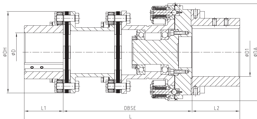
Bauart 00-1 bis 00-3 mit RADEX®-N
