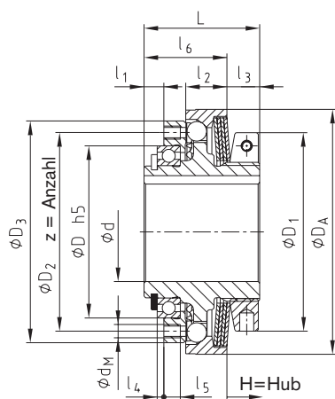
Nabenausführung 1.0 (Nutmachung nach DIN 6885)
