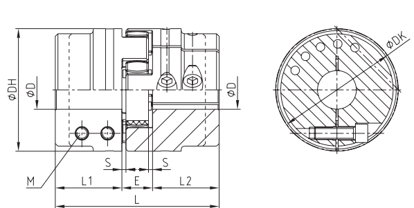
ROTEX® 38 - 90
