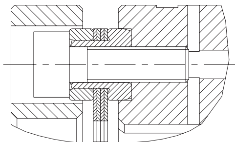
Gr. 5 bis 10 (zylindrische Buchse)
