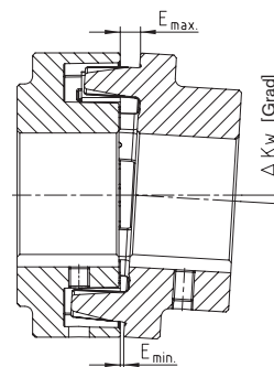
Winkelverlagerung ΔK w
