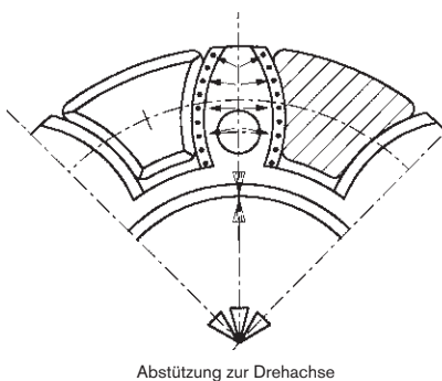
Begrenzung durch konkave Nockenform bei hoher Drehzahl/ Fliehkraft und Elastomervorspannung
