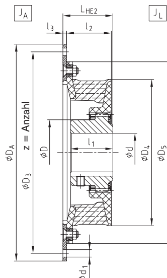
Bauart HE2
