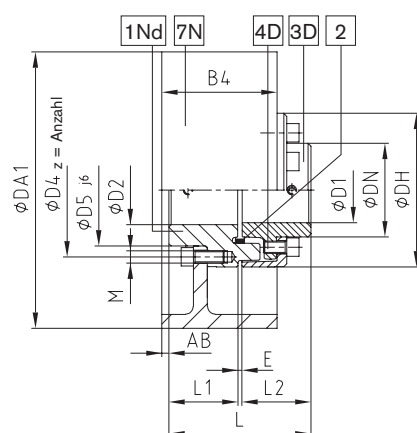
Bremstrommel Bauart ADR-BTA
