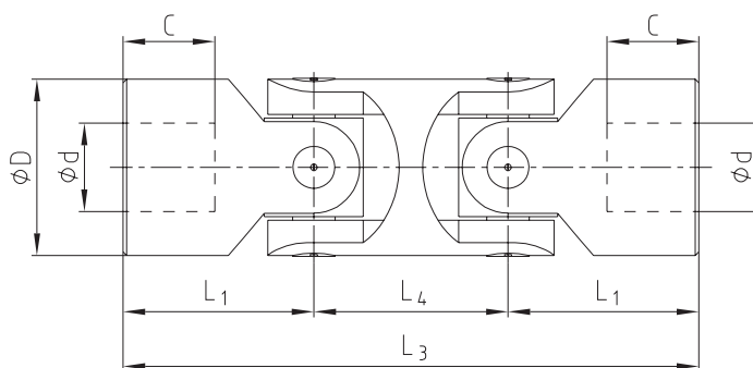
Präzisions-Doppelgelenk HD
