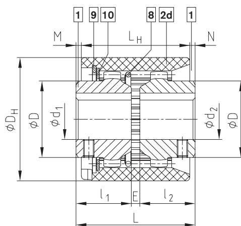
Bauart Spez.-I
