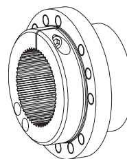
Ausf. 2.7 Klemmnabe: doppelt geschlitzt mit Profil
