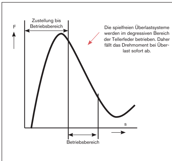
Federkennlinie
