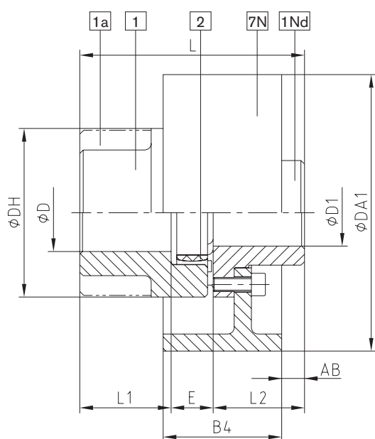
Bremstrommel Bauart BTAN
