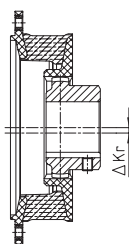
Radialversatz \Delta K_r
