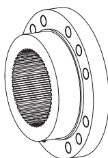
Ausf. 1.3 Nabe mit Profilverzahnung
