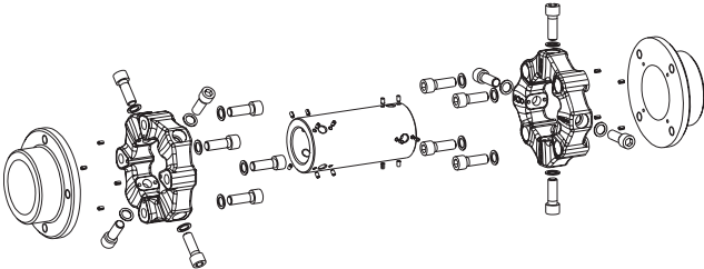
Größe 12 - 280
