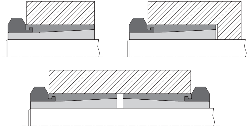
Anwendungsbeispiel Nabenform
