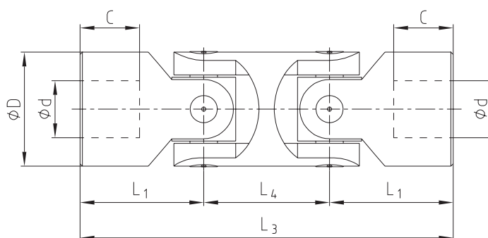
Präzisions-Doppelgelenk XD
