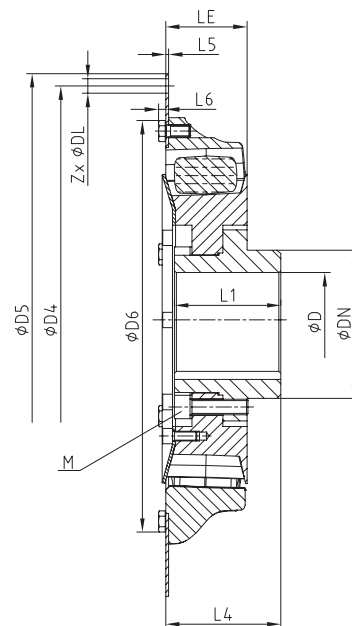
Ausführung B (adaptiver Flansanschluss)
