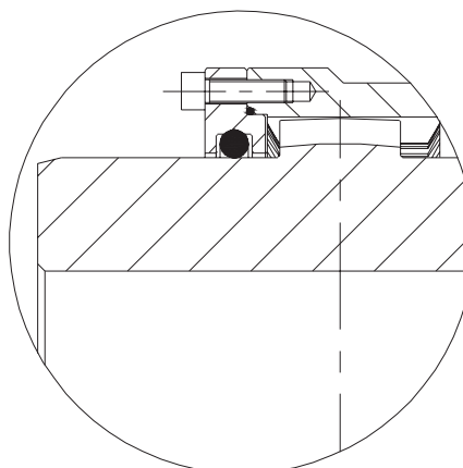
Bauart DR
