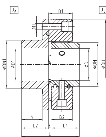
Größe 12 - 280
