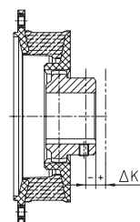
Axialversatz \Delta K_a
