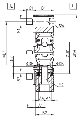
Größe 12 - 280
