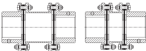
Bauart NANA 3 (s. Seite 182)
