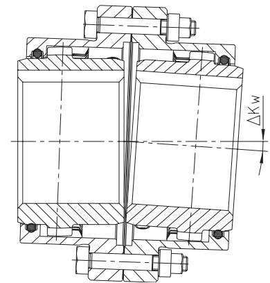
Winkelverlagerung
