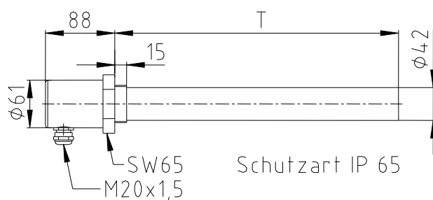
Bild 1: Type EHP - G 1 1/2" ohne Temperaturregler
