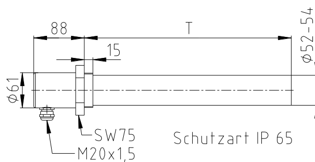
Bild 2: Type EHP - G 2" ohne Temperaturregler
