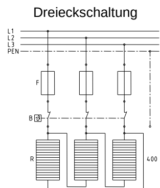
Bild 14: Schaltplan mit Thermostat - 400 V
