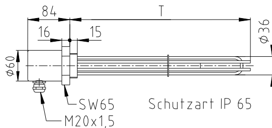
Bild 4: Type EH - G 1 1/2" ohne Temperaturregler
