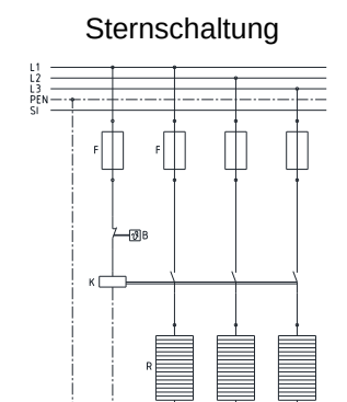
Bild 16: Schaltplan mit Thermostat > 400 V
