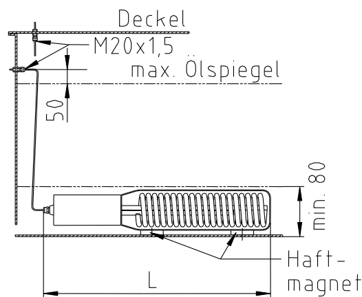
Bild 7: Einbauschema - TEHM
