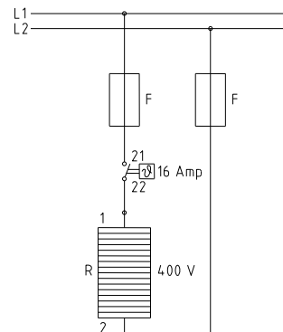
Bild 10: Schaltplan mit Thermostat - 400 V
