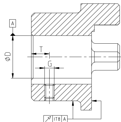
Bild 7: Rund- und Planlaufgenauigkeit
