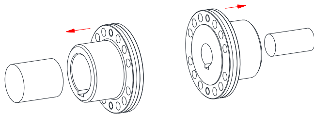
Bild 8: Montage der Kupplungsflansche
