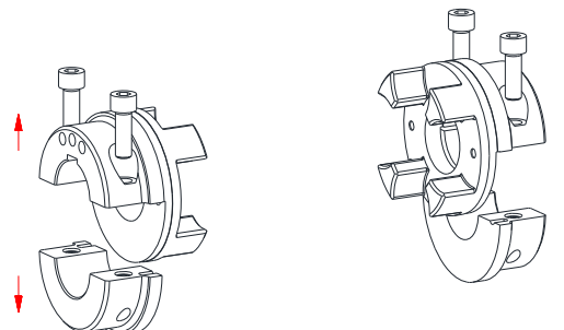
Bild 11: Demontage der Halbschalen
