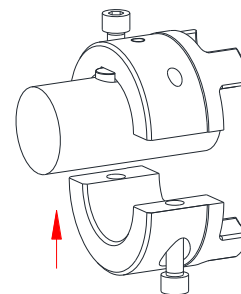
Bild 16: Montage der SPLIT-Nabe auf die Welle
