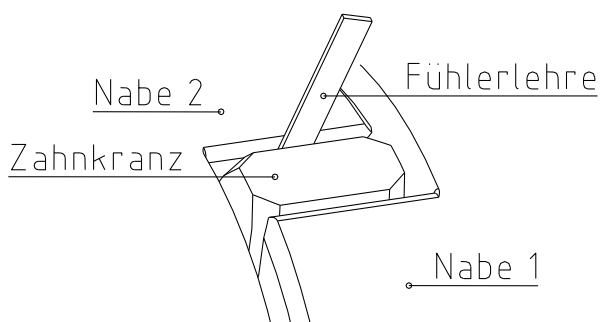
Bild 23: Überprüfung der Verschleißgrenze
