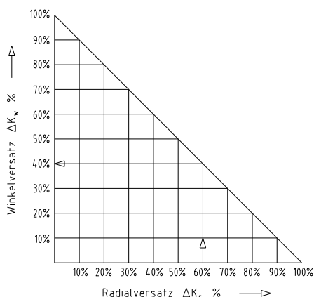
Winkelverlagerungen
