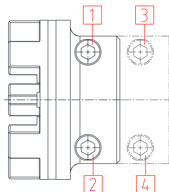
Bild 14: Anziehen der Schrauben
