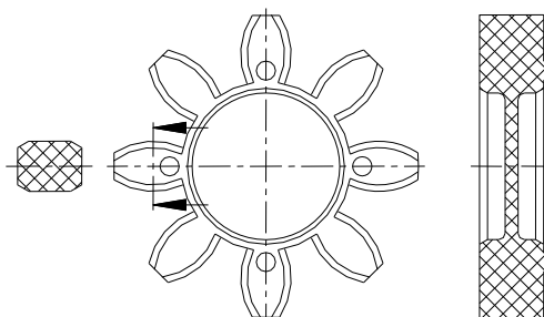
Bild 22: ROTEX® GS-Zahnkranz
