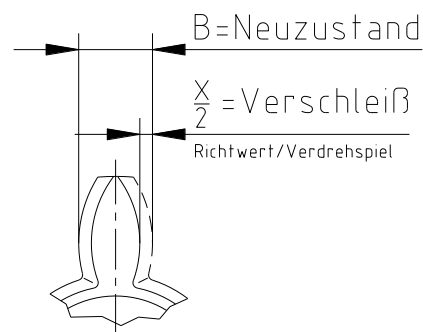
Bild 24: Zahnkranzverschleiß
