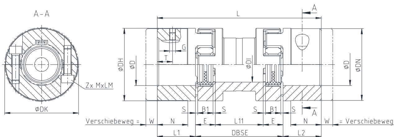
Bild 3: ROTEX® Bauart ZS-DKM-SH
