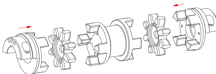
Bild 12: Montage der Nabengrundkörper, Zahnkränze und DKM-H-Mittelstück
