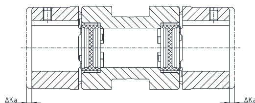
Axialverlagerungen
