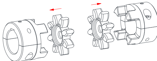
Bild 17: Montage der Zahnkränze
