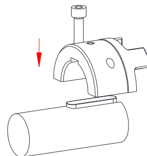
Bild 15: Montage der Halbschale
