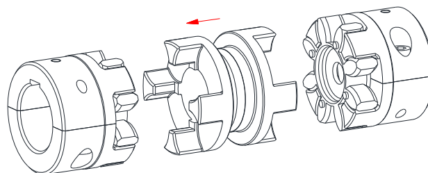
Bild 18: Montage des DKM-H-Mittelstückes
