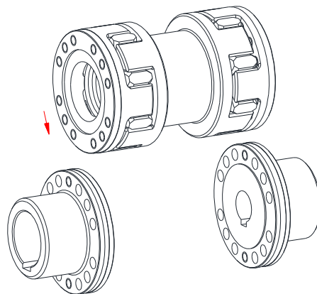
Bild 10: Montage der Baugruppe
