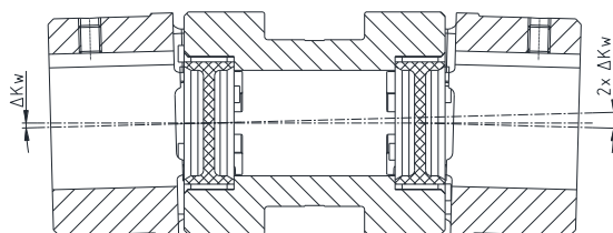
Winkelverlagerungen
