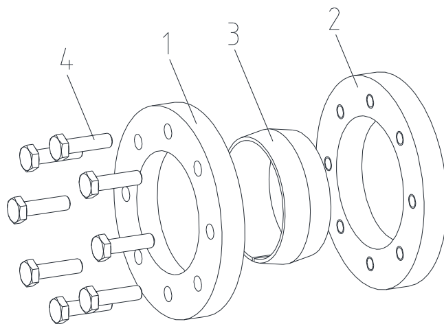
Bild 3: Bauteile des Spannsatzes
