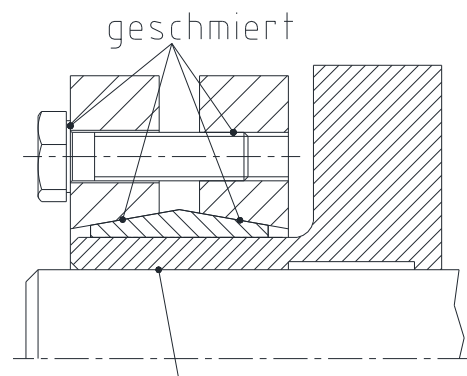
Bild 4: Reinigen/Fetten der Flächen
