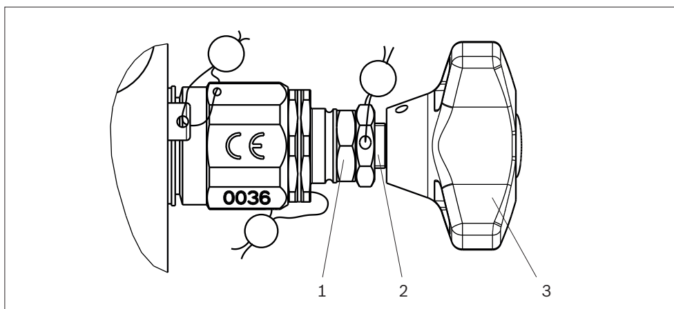
Fig. 1: Desserrage du contre-écrou
