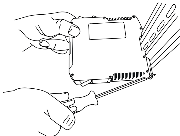
Abb. 6: Demontage des VT-MRPA1-2X von der Hutschiene
