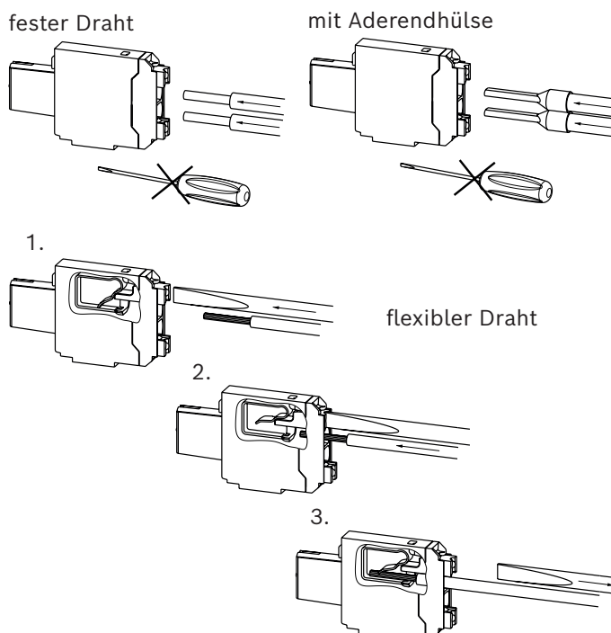
Abb. 3: „PUSH-IN“-Kontakt
