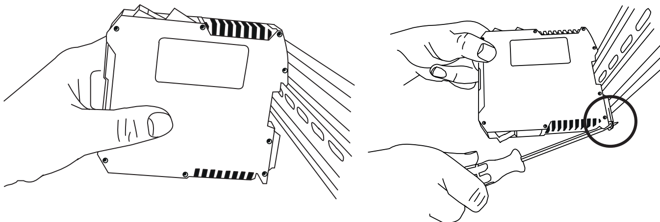
Abb. 1: Montage des VT-MRPA1-2X auf Hutschiene
