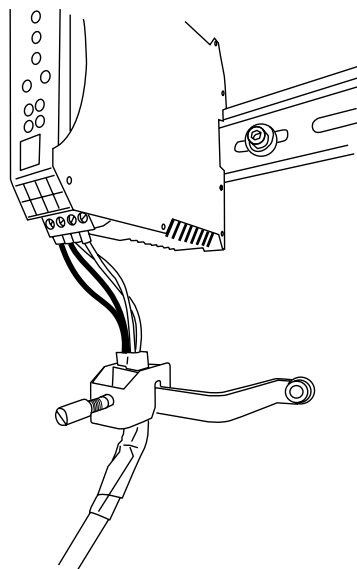
Abb. 2: Schirmung des VT-MRPA1-2X
