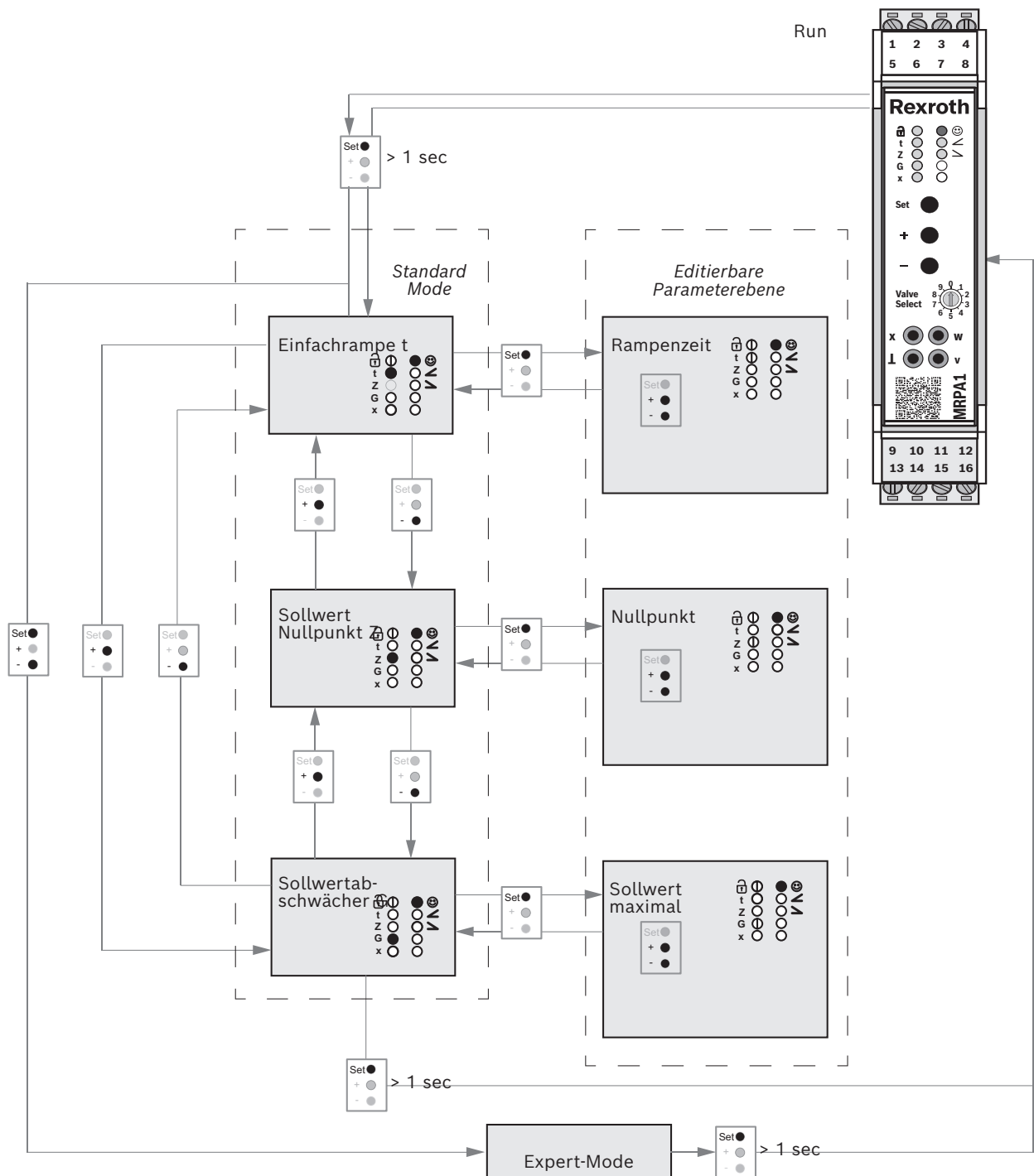
Abb. 5: Menüstruktur
